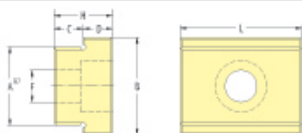
GRUPPO VITE/SCREW UNIT ED03
