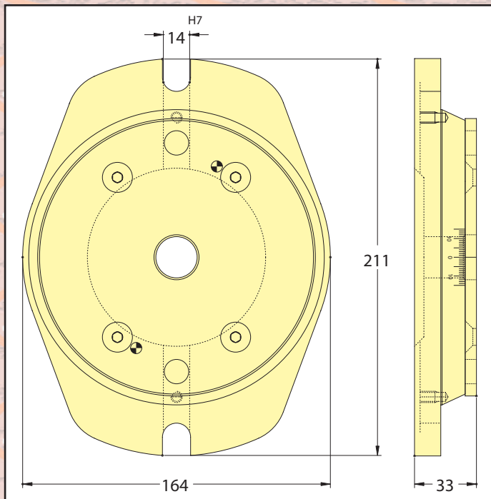
GANASCIA A V/V-JAW GP. 76
