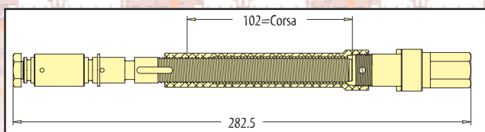
GRUPPO VITE/SCREW UNIT GP. 76
