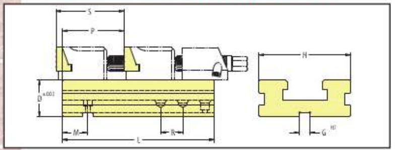
PROLUNGA FISSA/FIXED EXTENSION SPE. 81
